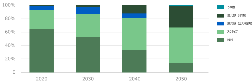
グラフ6：2022年度1.5℃シナリオの鉄源別粗鋼生産割合
