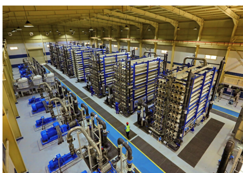
エジプト Al Yosr 海水淡水化施設
